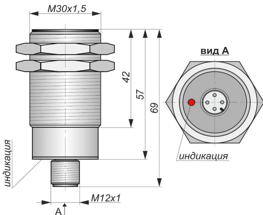
Габаритный чертеж
